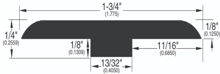
T-Mold (281018)
